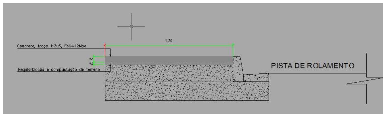
Figura 1 – Componentes da estrutura do passeio.
